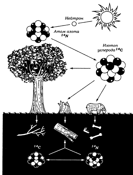
Схема радиоуглеродного метода
