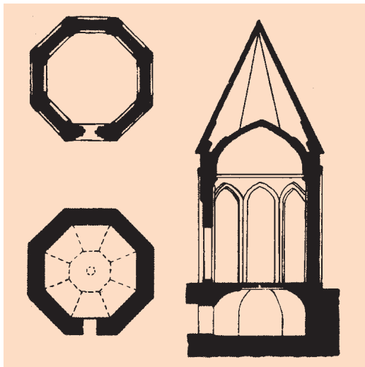
Türbənin planı və kəsiyi.
