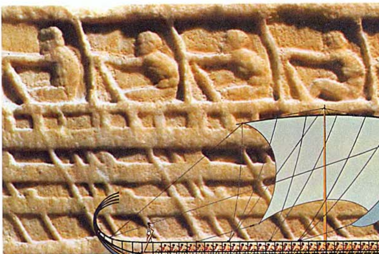
Древнегреческий рельеф, на котором изображен фрагмент триеры с гребцами, и современный рисунок триеры
